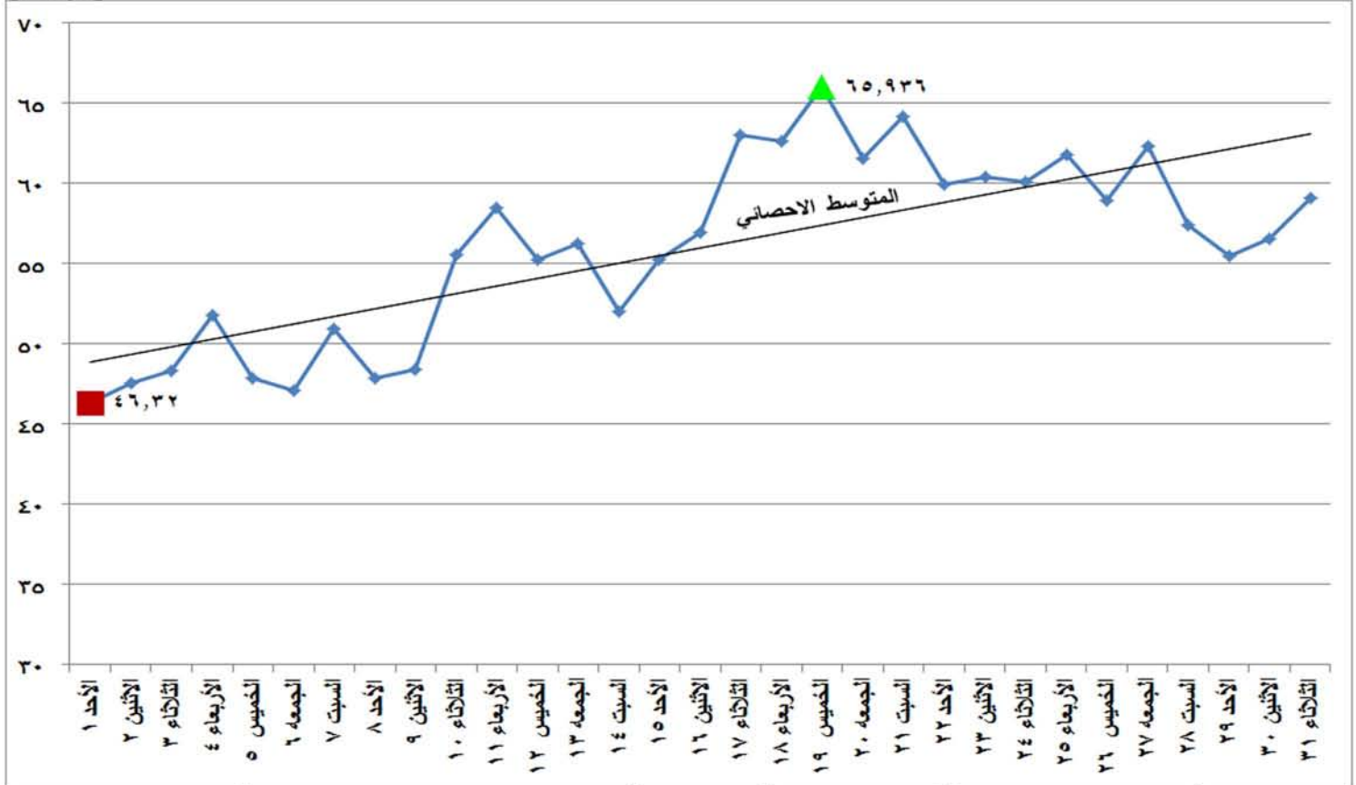
شكل (٢١) الطاقة الكهربائية المنتجة من المصادر غير الحرارية خلال شهر مايو ٢٠١٦
