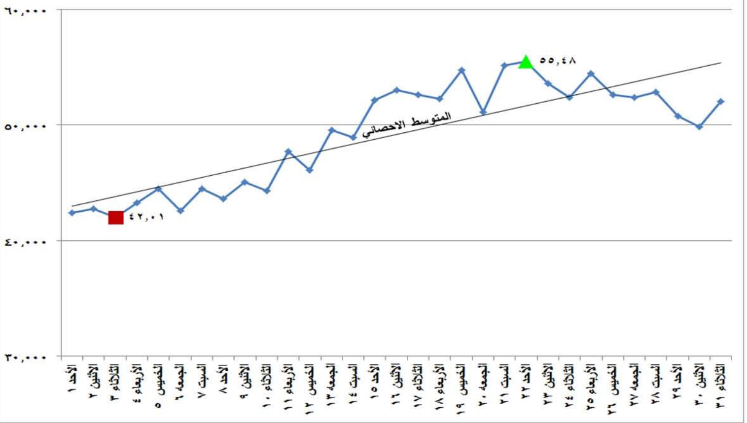
شكل (٢٣) الطاقة الكهربائية المنتجة من المصادر المائية خلال شهر مايو ٢٠١٦
