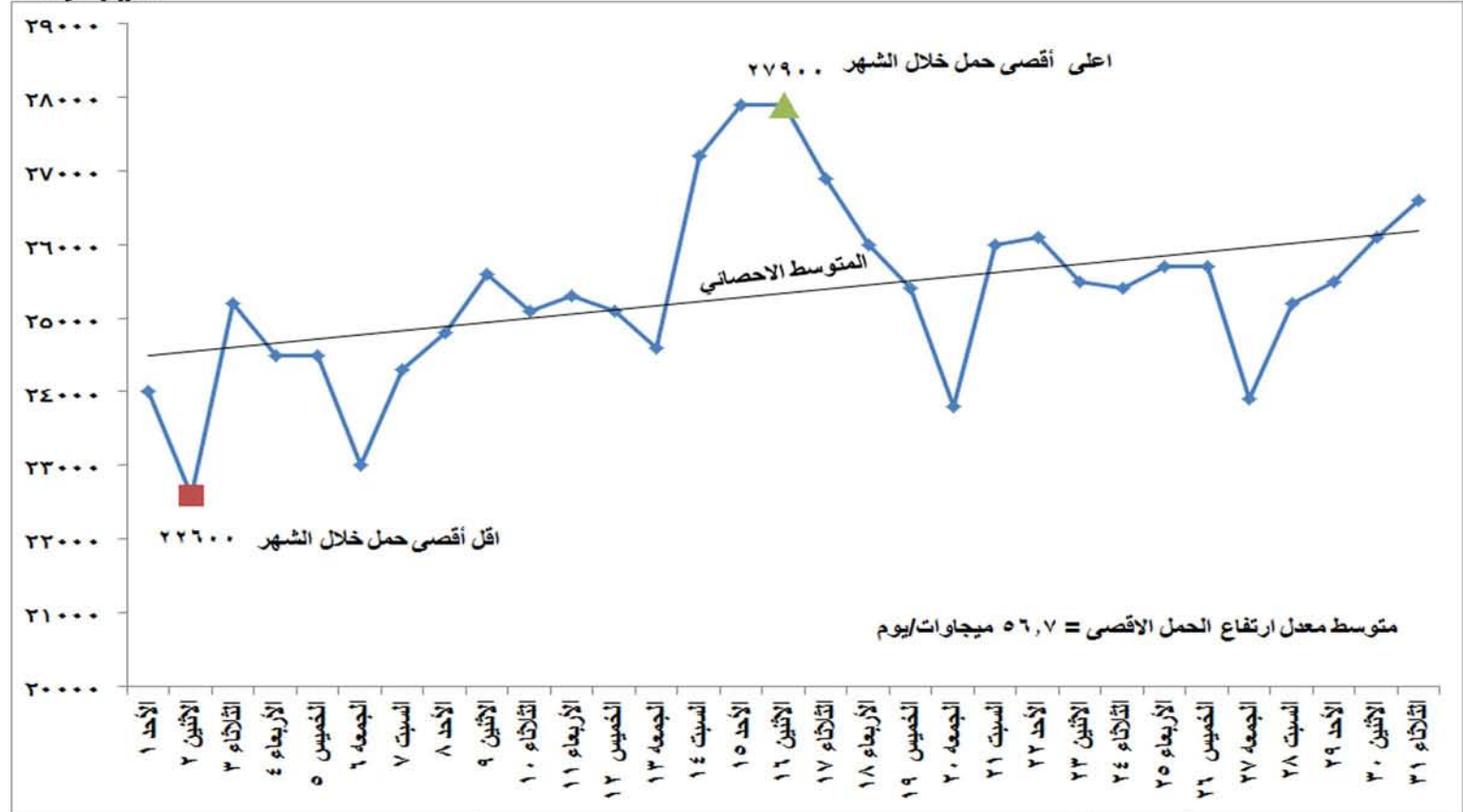
شكل (١) تطور الحمل الاقصى اليومي خلال شهر مايو ٢٠١٦
