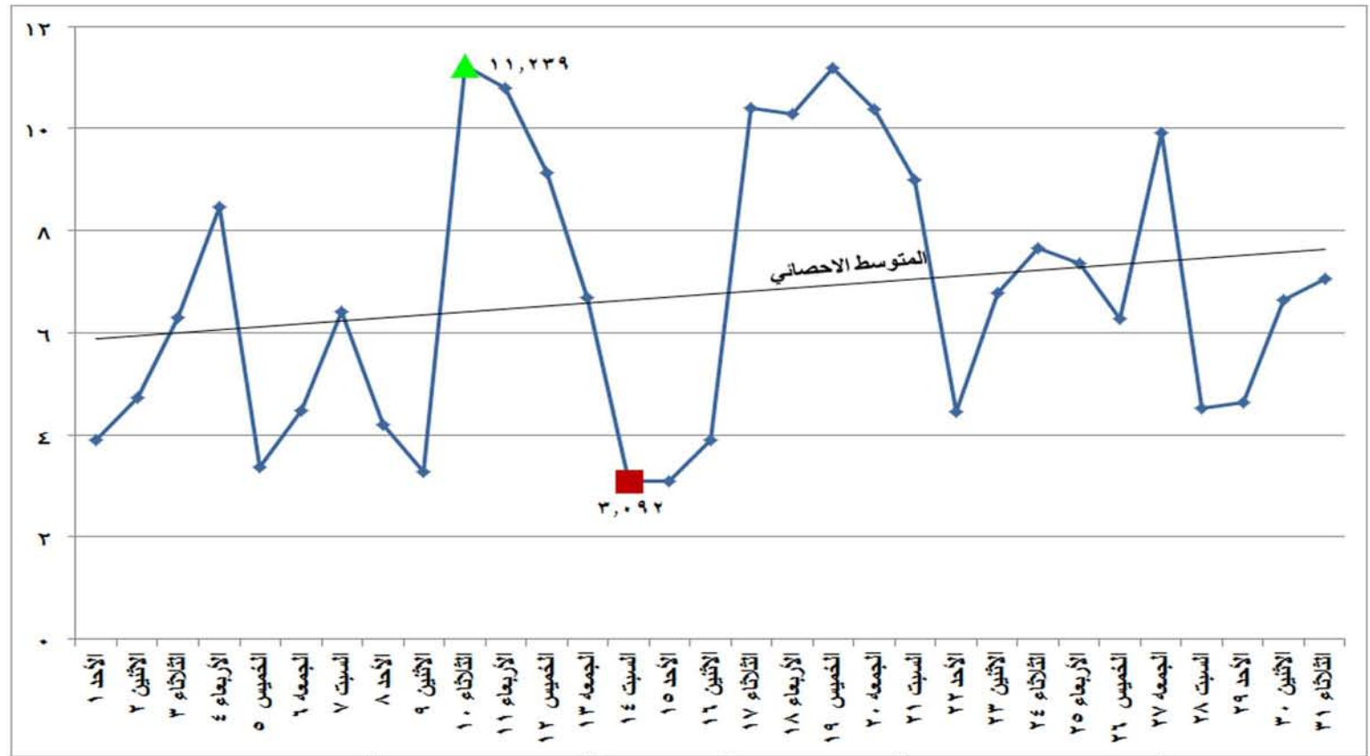
شكل (٢٥) الطاقة الكهربائية المنتجة من الرياح والشمس خلال شهر مايو ٢٠١٦
