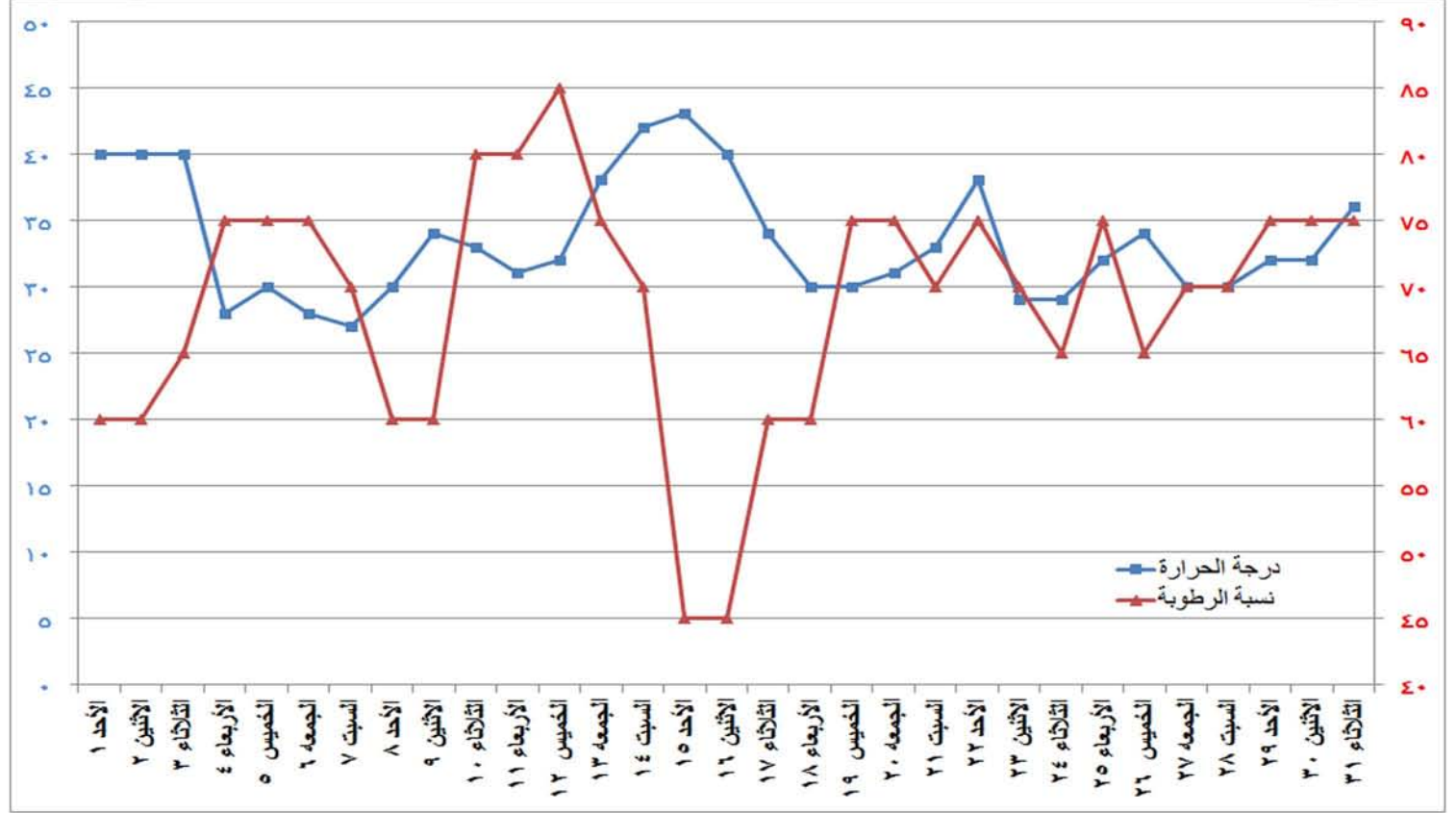
شكل (١١) التغيير في درجة الحرارة والرطوبة النسبية خلال شهر مايو ٢٠١٦
