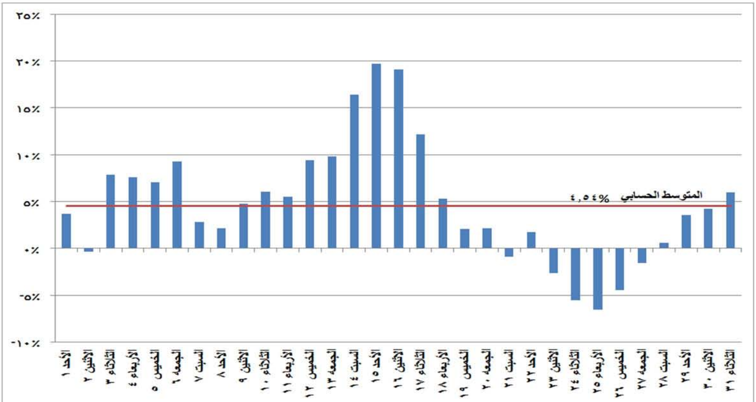
شكل (١٦) نسب التغير في الطاقة الكهربائية المنتجة خلال شهر مايو ٢٠١٦ مقارنة بالشهر المماثل من العام السابق
