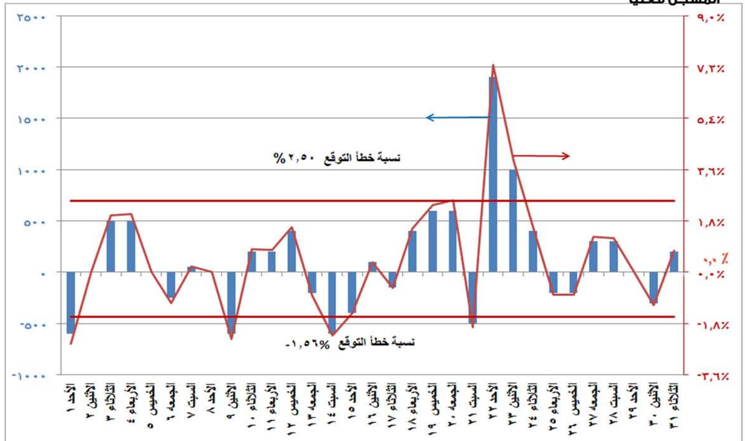
شكل (١٠) الفرق بين الحمل الأقصى المتوقع والمسجل فعليا ونسبة الفرق إلى الحمل المسجل فعليا خلال شهر مايو ٢٠١٦
