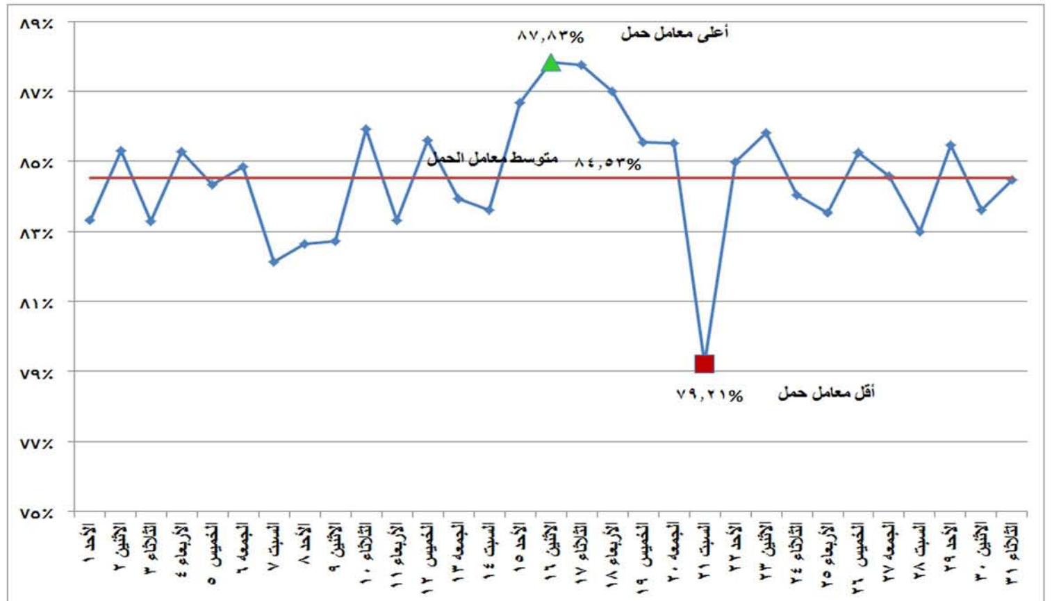
شكل (١٢) إجمالي معامل الحمل لوحدات الانتاج خلال شهر مايو ٢٠١٦
