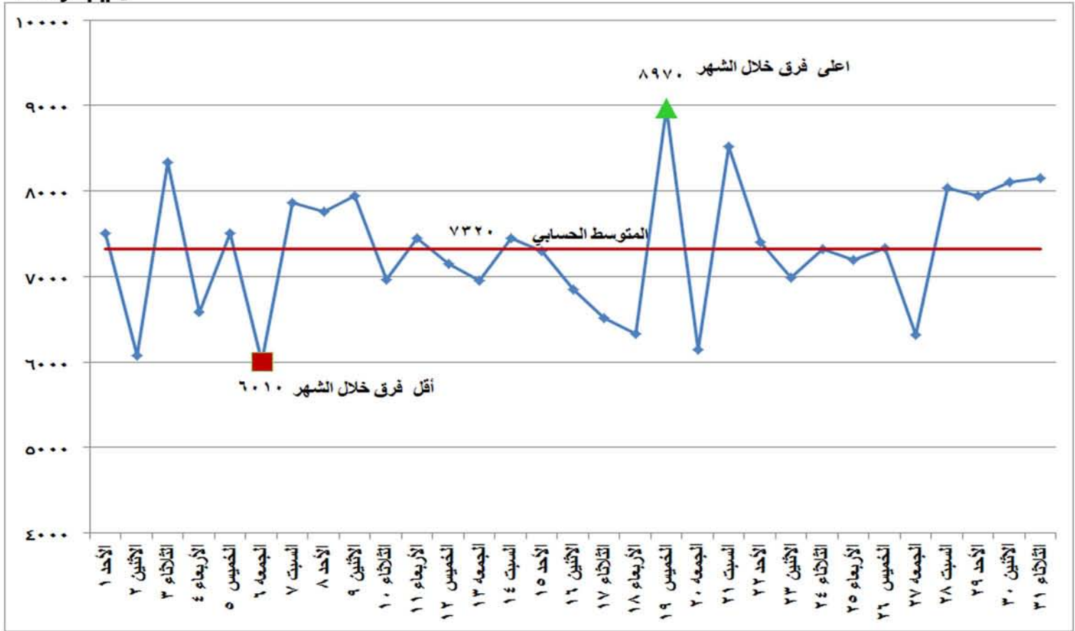
شكل (٣) الفرق بين أقصى وأدنى حمل خلال شهر مايو ٢٠١٦
