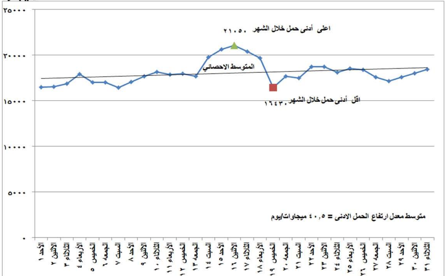
شكل (٢) تطور الحمل الادنى اليومي خلال شهر مايو ٢٠١٦
