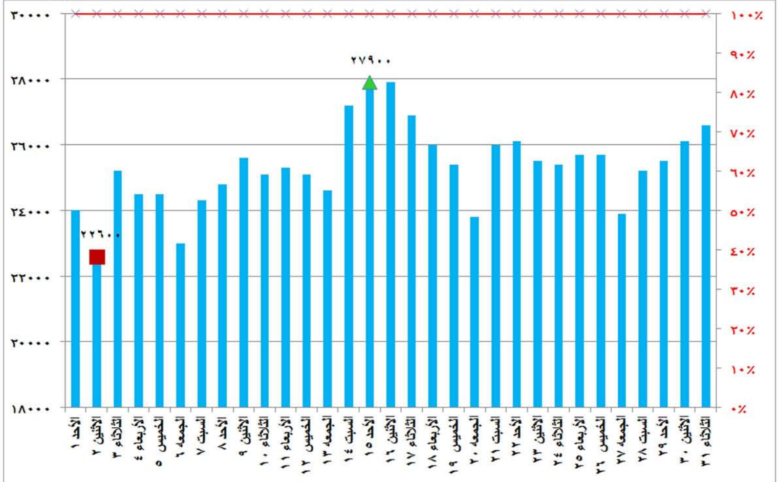
شكل (٥) قدرات الانتاج المتاحة ونسبتها للحمل الاقصى خلال شهر مايو ٢٠١٦
