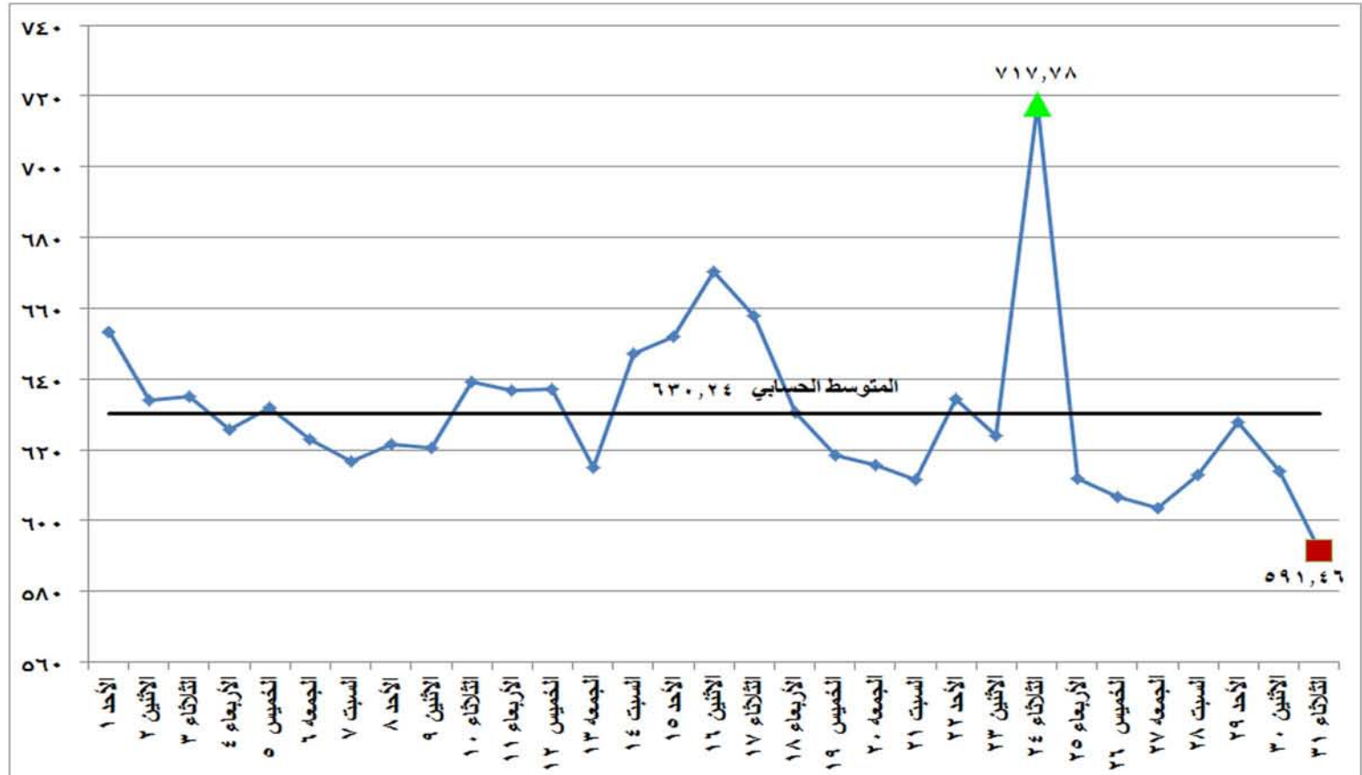
شكل (١٤) معامل انبعاثات غاز ثاني اكسيد الكربون المكافئ على مدى شهر مايو ٢٠١٦
