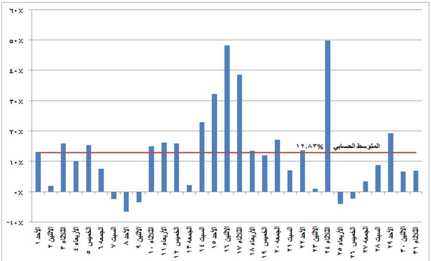
شكل (٢٠) نسب التغير في استخدام المازوت في إنتاج الطاقة الكهربائية خلال شهر مايو ٢٠١٦ مقارنة بالشهر المماثل من العام السابق
