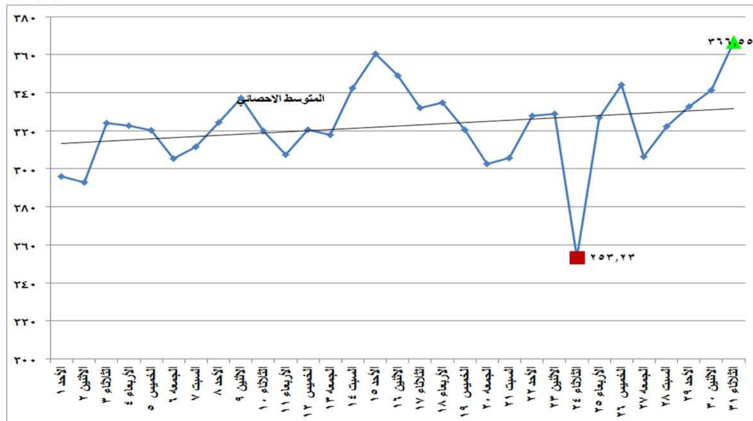
شكل (١٧) الطاقة الكهربائية المنتجة من الغاز الطبيعي خلال شهر مايو ٢٠١٦
