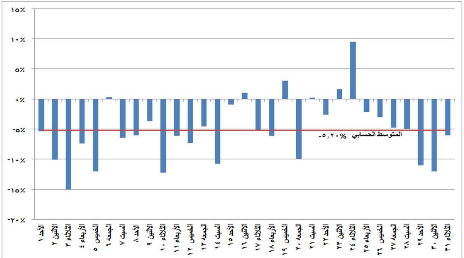
شكل (٢٤) نسب التغير في استخدام المصادر المائية في إنتاج الطاقة الكهربائية خلال شهر مايو ٢٠١٦ مقارنة بالشهر المماثل من العام السابق
